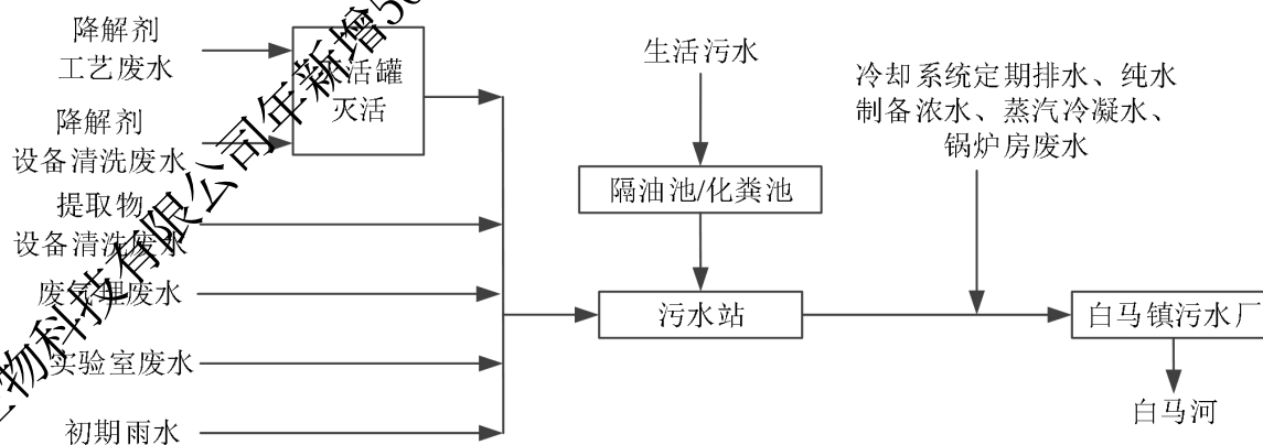
图 6.3-1 拟建项目废水处置走向示意图
