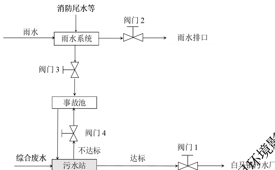
图 6.7-2 事故废水防范和处理流程示意图
