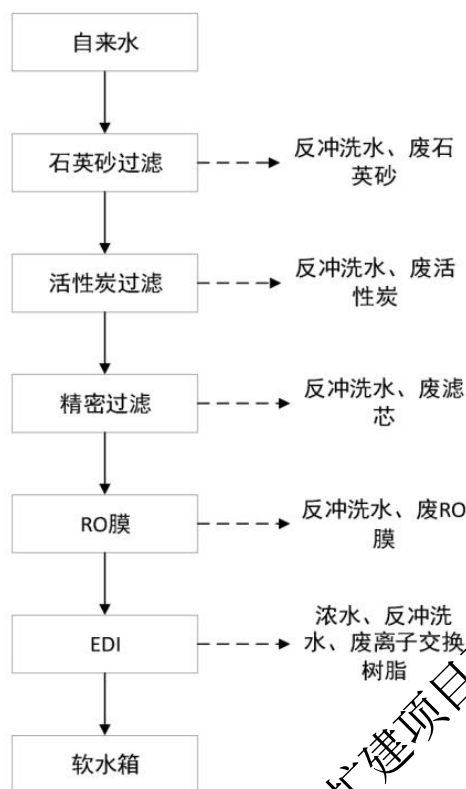
图 3.2-3 软水制备系统流程图示意图
