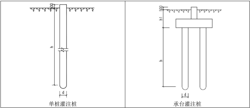
图 3.1-1 本项目塔基基础一览图
