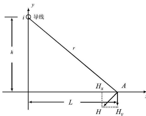
图 6.1-7 磁场向量图
