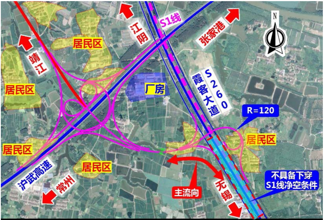
图 2-1-12 徐霞客枢纽互通和徐霞客互通平面布置示意图
