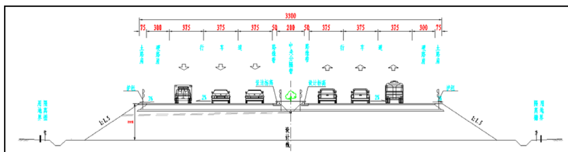
图 2-1-7 双向六车道路基标准横断面示意图
