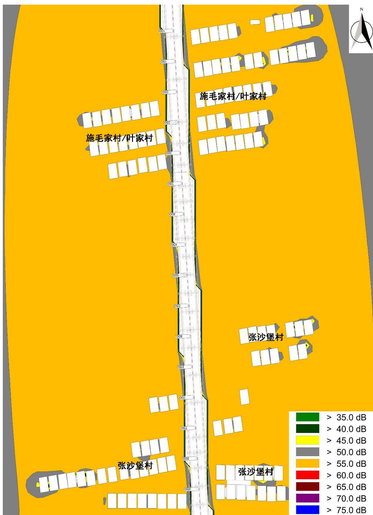
图 4-1-4 K0+000-K0+800 运营近期昼间水平方向等声级线图 H=4.2m
