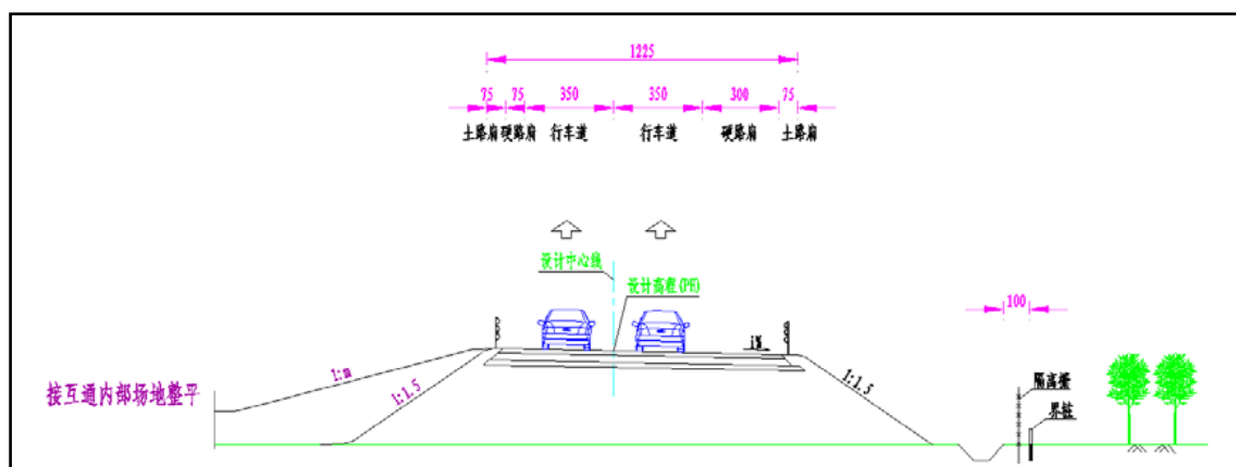
图 2-1-4 单向双车道匝道路基标准横断面 I 示意图
