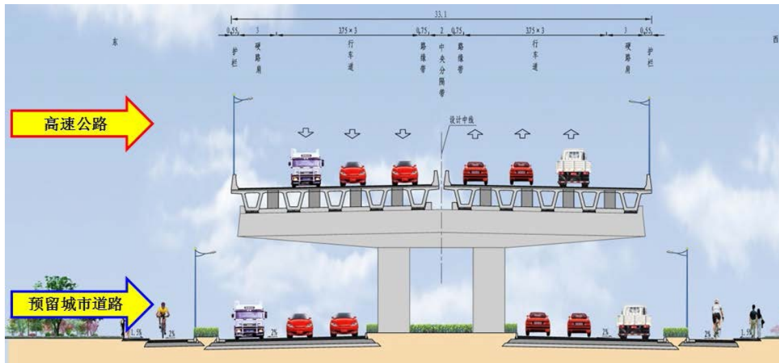
图 2-1-1 规划城镇路段标准横断面布置示意图
