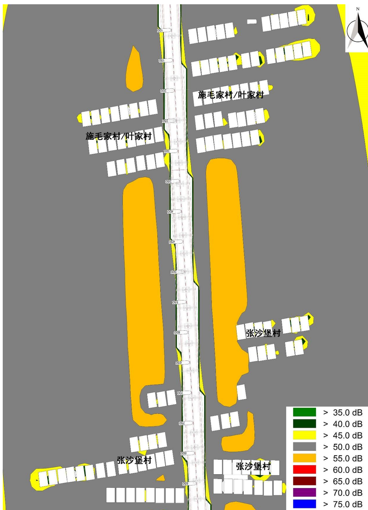
图 4-1-9 K0+000-K0+800 运营远期夜间水平方向等声级线图 H=4.2m
