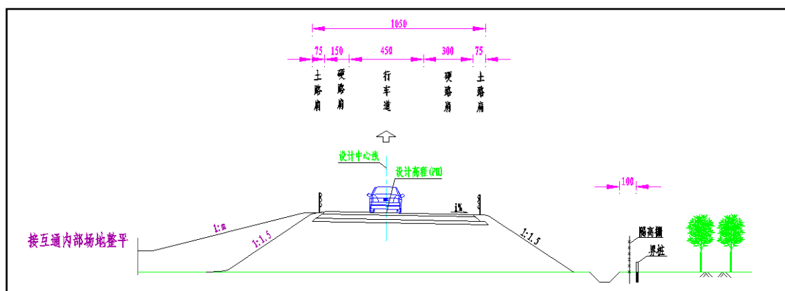
图 2-1-3 单向单车道匝道路基标准横断面示意图
