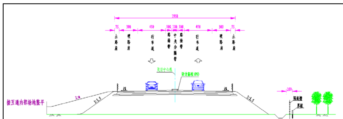
图 2-1-6 对向分隔式双车道匝道路基标准横断面示意图
