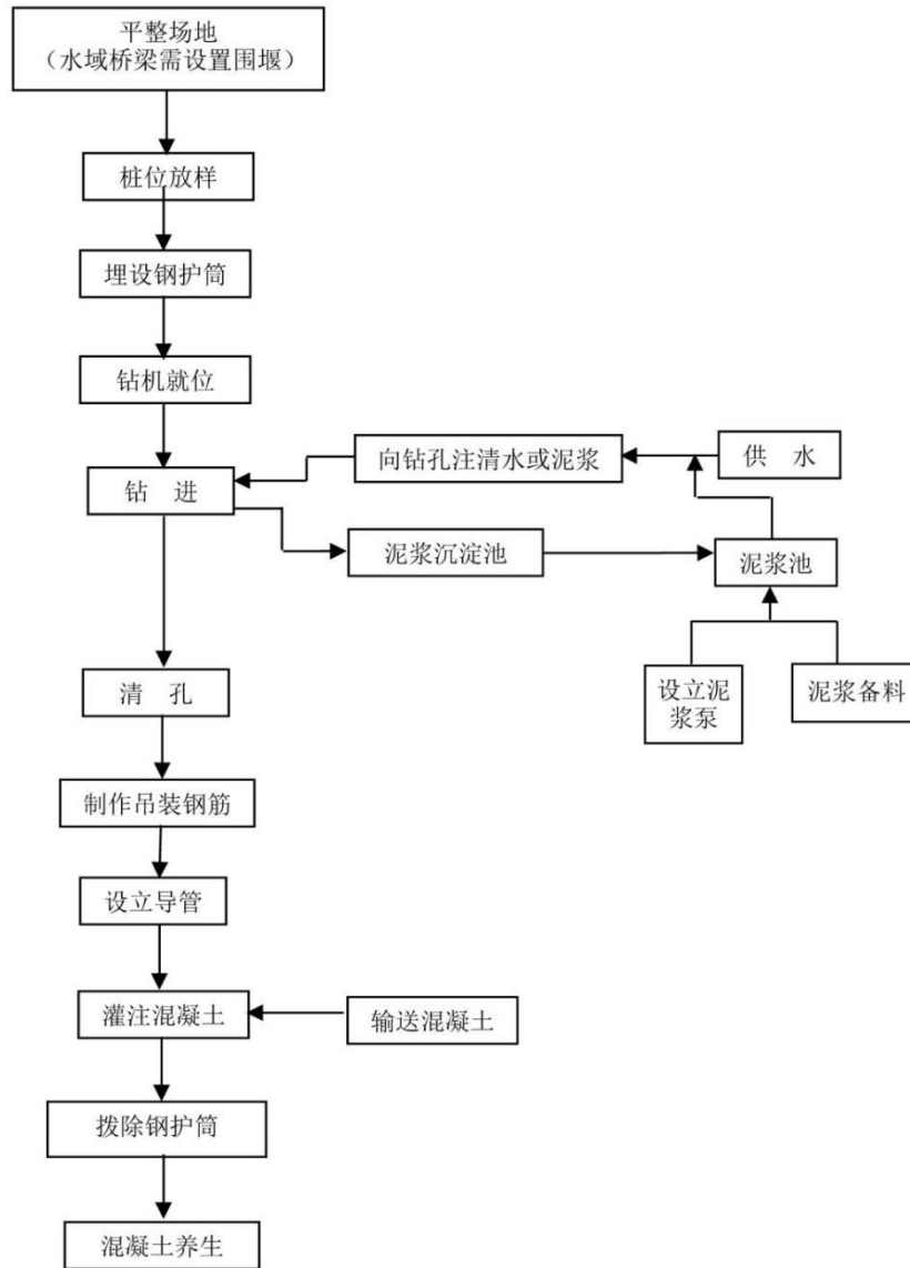
图 2-1-13 典型桥梁施工工艺流程示意图
