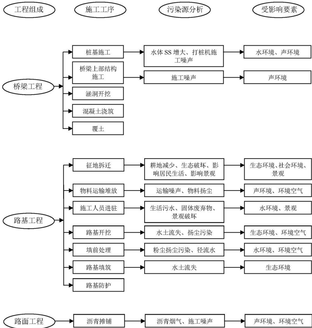
图 5-1-1 施工期污染源分析示意图
