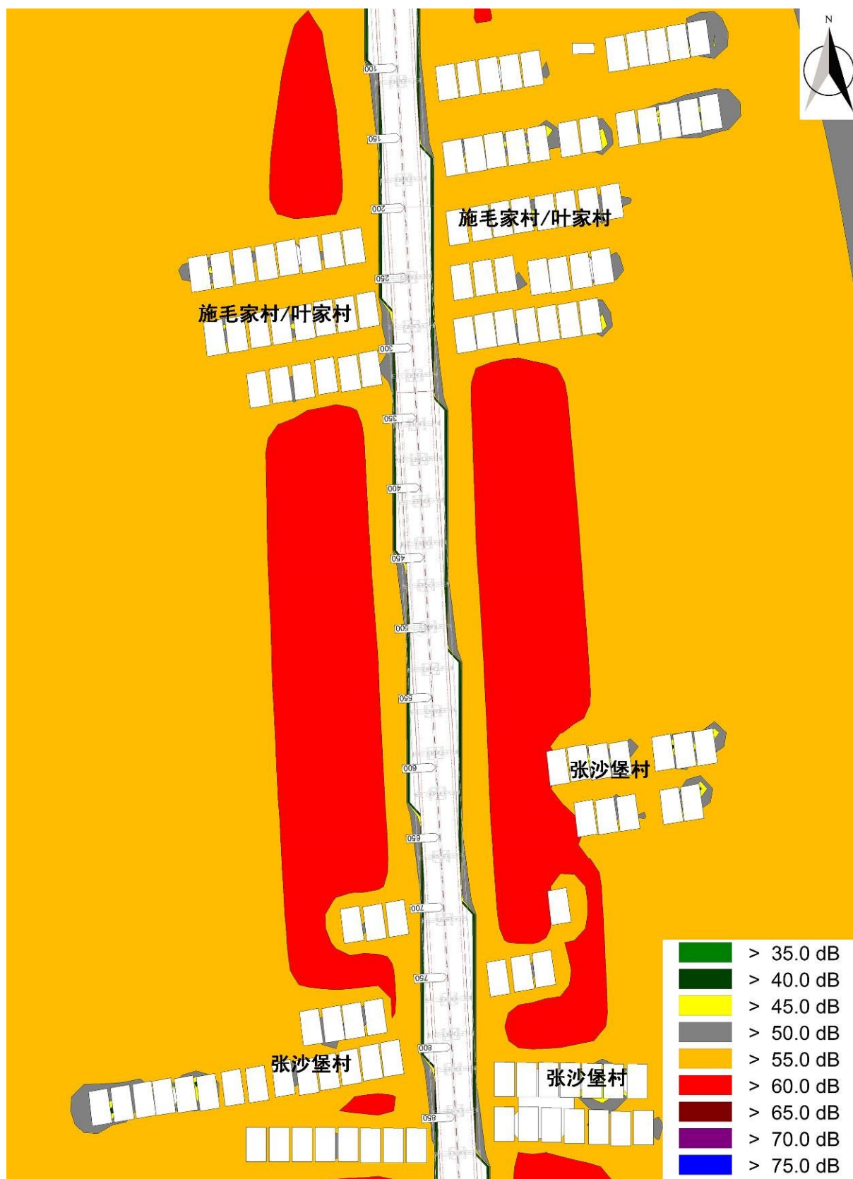
图 4-1-6 K0+000-K0+800 运营中期昼间水平方向等声级线图 H=4.2m
