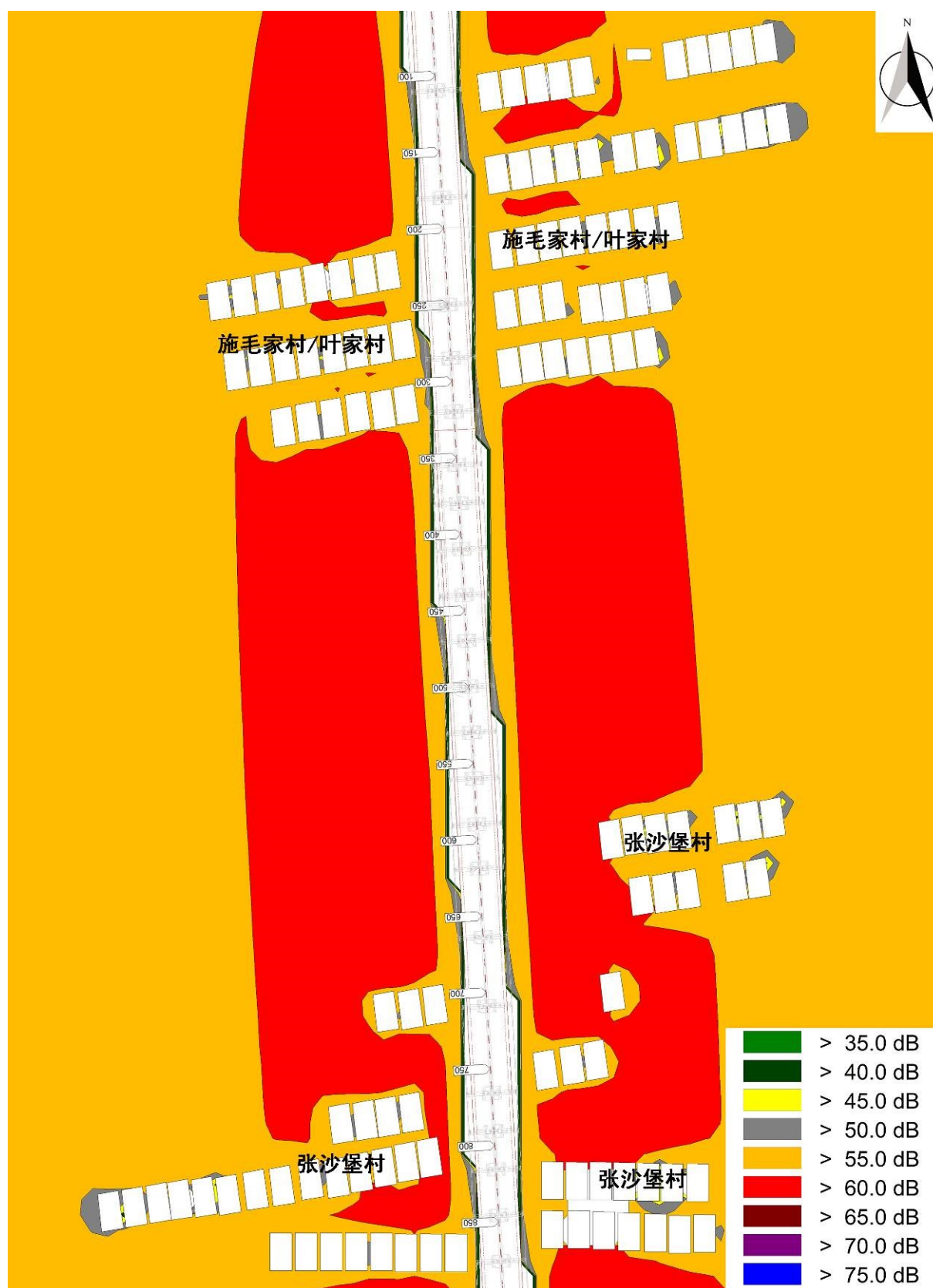
图 4-1-8 K0+000-K0+800 运营远期昼间水平方向等声级线图 H=4.2m
