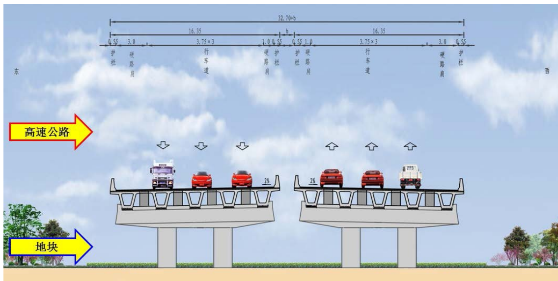
图 2-1-2 非规划城镇段标准横断面布置示意图
