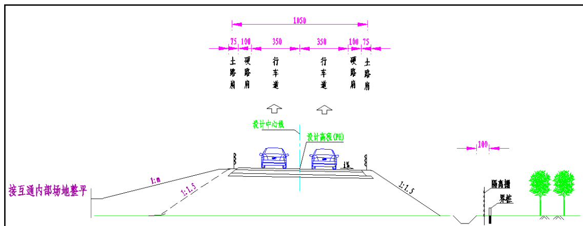
图 2-1-5 单向双车道匝道路基标准横断面 II 示意图
