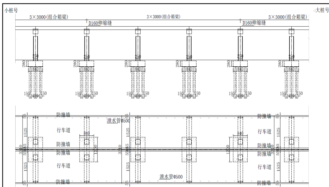
图 2-1-9 标准段桥梁立面和平面布置示意图
