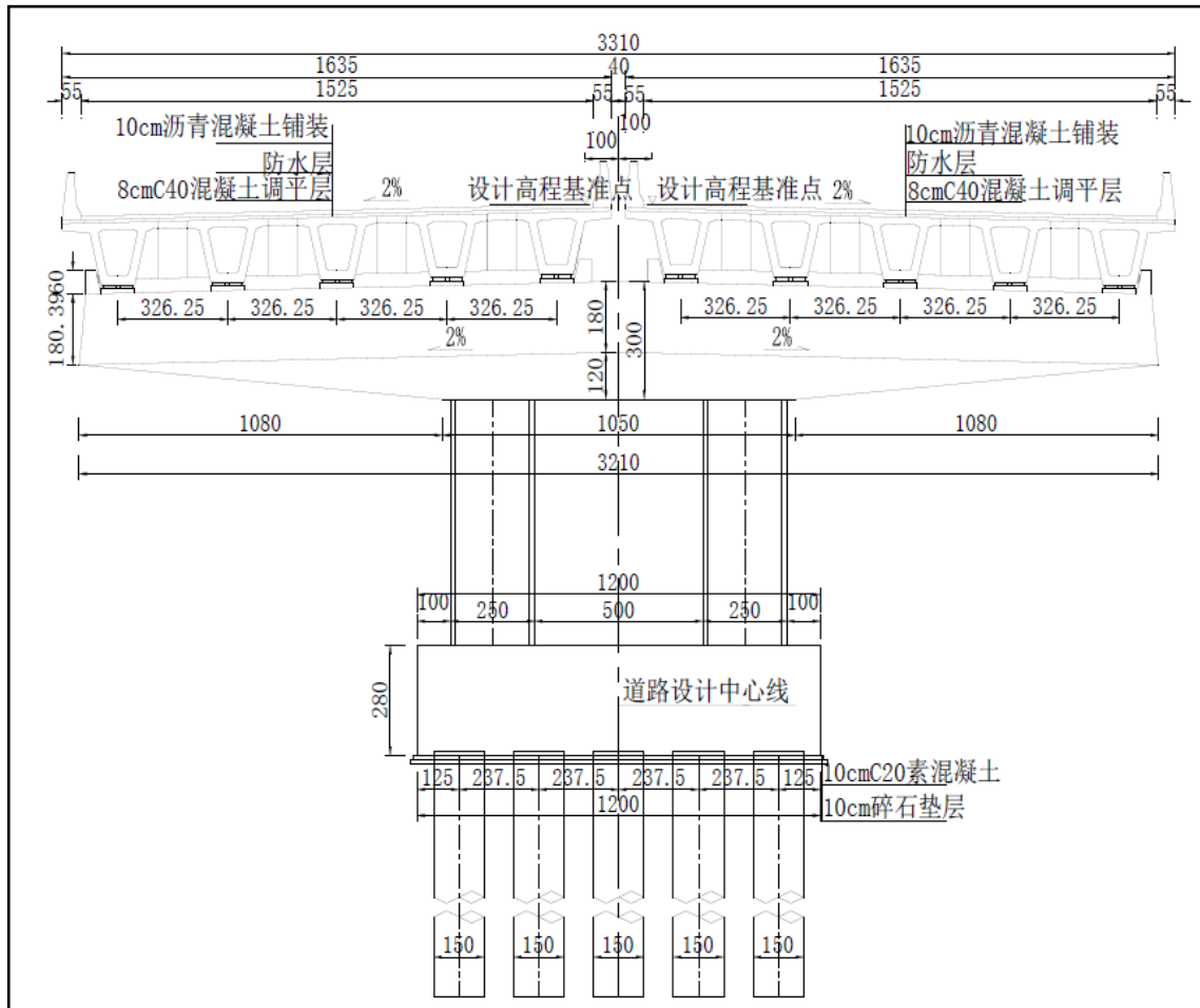
图 2-1-10 标准桥梁横断面布置示意图
